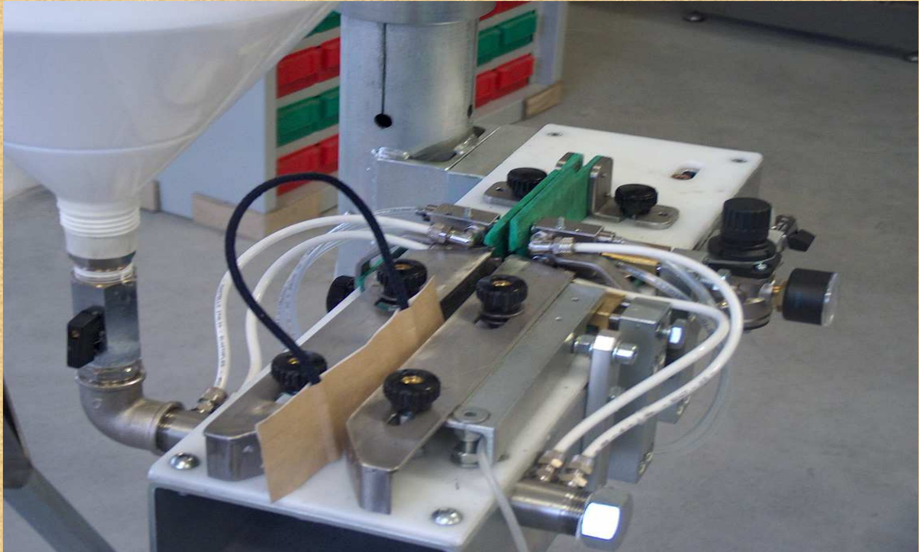
Foto del Banco di lavoro dell'Incollatore Automatico di Maniglie da applicare a mano su Sacchi di Lusso. Photo of the Workbench of Automatic gluing handles applied by hand on Luxury Bags.
