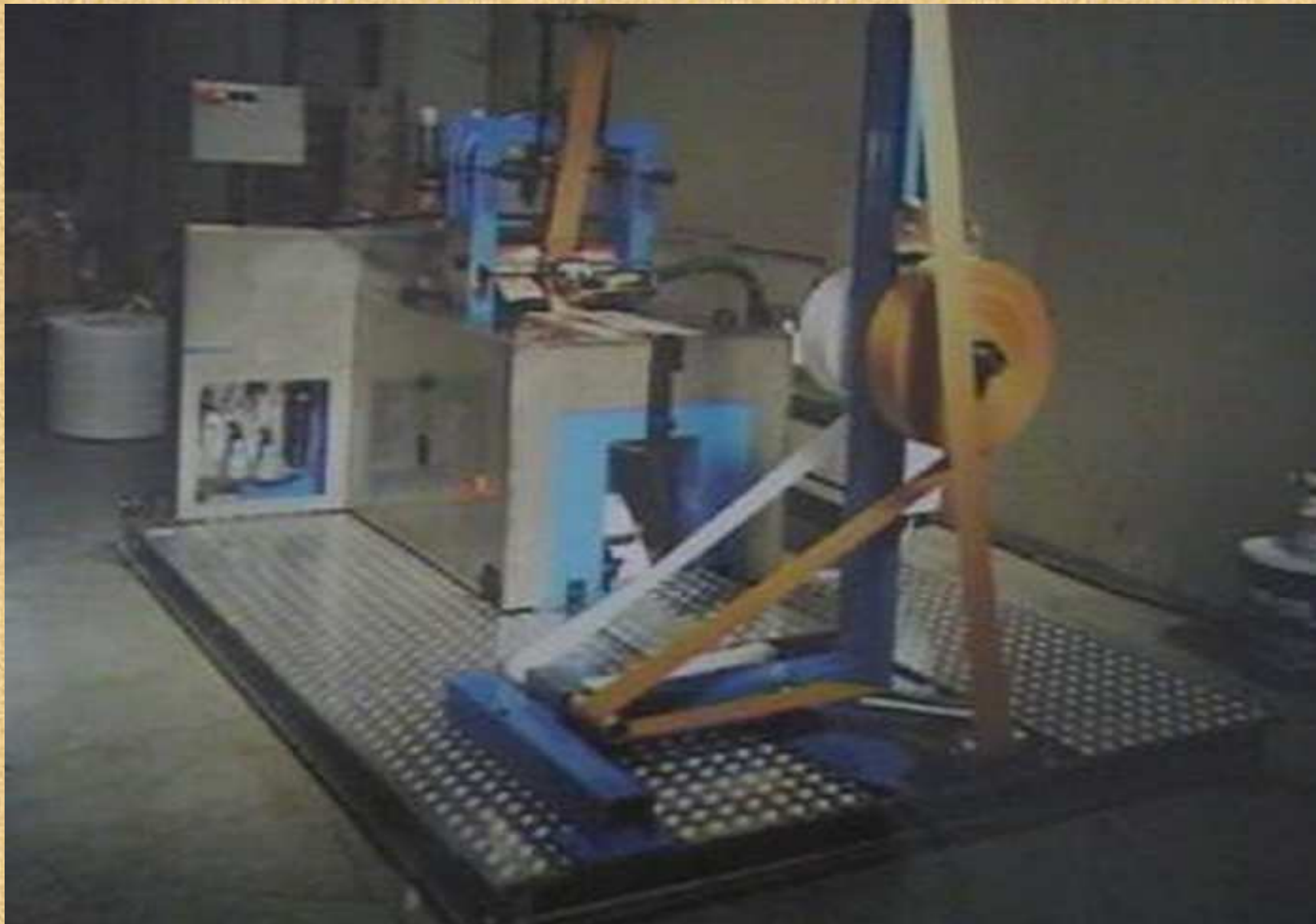
Manigliatrice per Maniglie di Carta Sfuse di Taglia: MINI e MEDIUM Paper Free Handles Making Machine Size: MINI and MEDIUM
